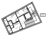
planta sótano
